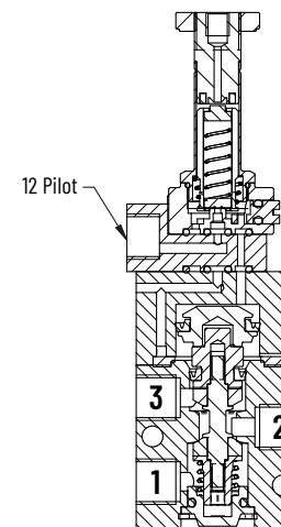
SEZIONE A-A
