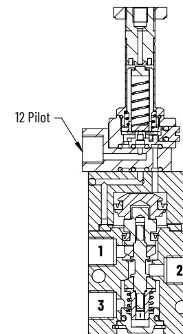
SEZIONE A-A
