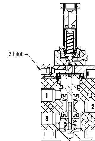
SEZIONE A-A
