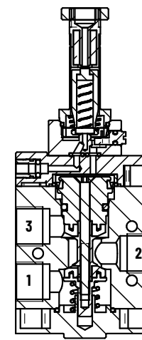
SEZIONE A-A
