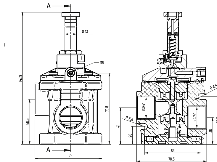
SEZIONE A-A
