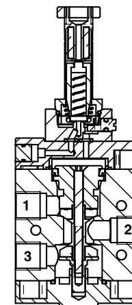
SEZIONE A-A
