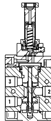
SEZIONE A-A
