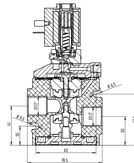
SEZIONE A-A
