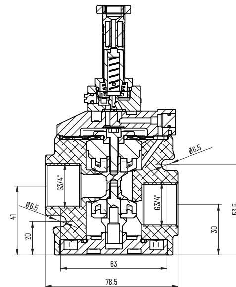
SEZIONE A-A
