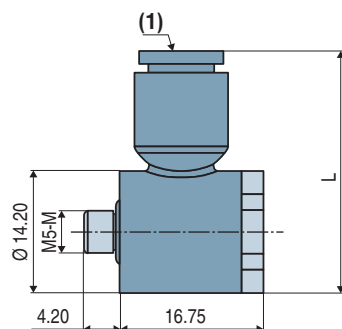
(1) Raccord instantané
